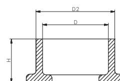
Demontagewerkzeug Disassembling Tool
