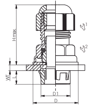
Demontagewerkzeug Disassembling Tool
