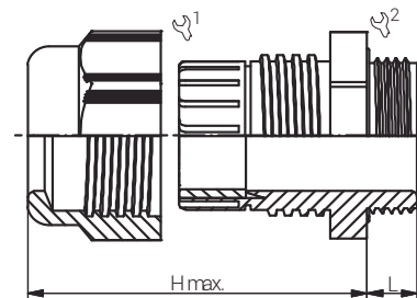
Polyamid Polyamide
