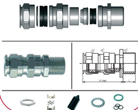
Kabelverschraubungen Ex e/d
