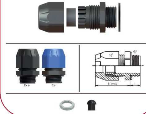
Kabelverschraubungen Ex e/i
